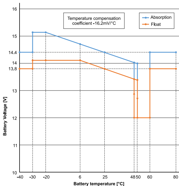
Temperatuur gecompenseerde laadgrafiek
